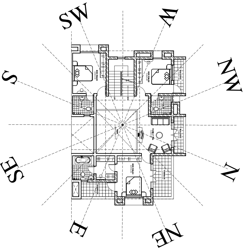
FIRST FLOOR PLAN (BUNGLOW 01)
